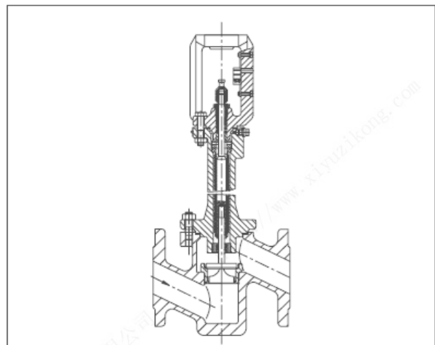
图 6 · 3241-1 型控制阀、锻钢类型 NPS ½ 至 3 配波纹管密封
