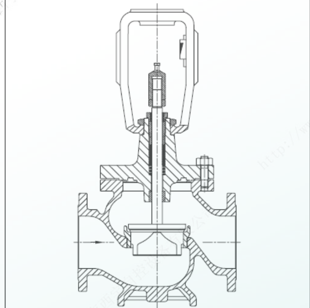
图 7 · 3241 型控制阀、NPS 8 至 12
