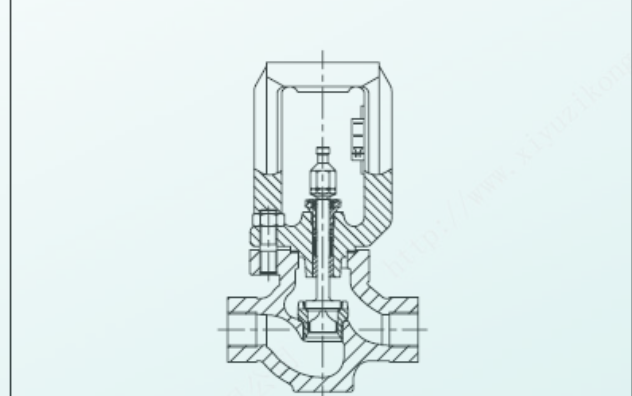
图 8 · 3241 型控制阀、NPS ½ 至 2 配 NPT 螺纹
