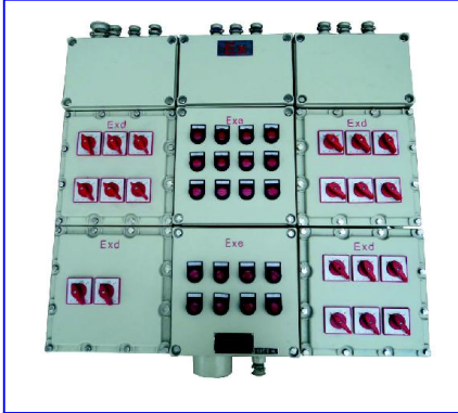
BXM(D) 51系列防爆照明（动力）配电箱（IIB）
