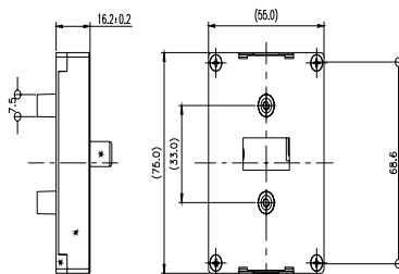
图 2-3 键盘盒的外形及安装尺寸
