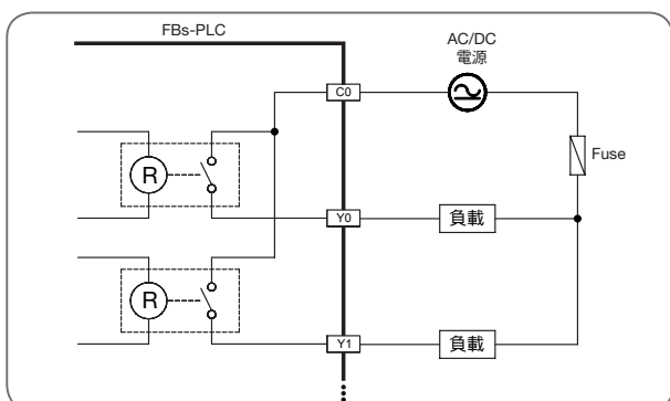
單端共點繼電器輸出接線
