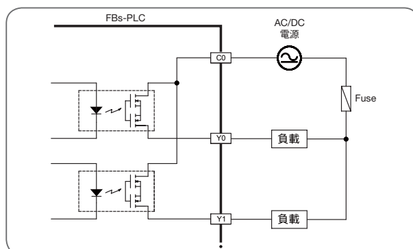
單端共點PhotoMOS輸出接線
