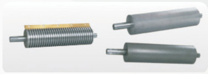
Roller type Optional flat spot roller, web roller and groove roller to meet different coating demand. 最常用滾輪分別為點狀、網狀、凹槽，可根據過膠的黏度和作用，選擇不同型號的滾輪塗佈
