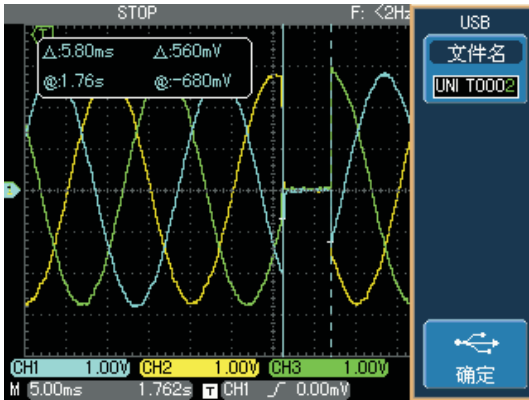
同相环境
