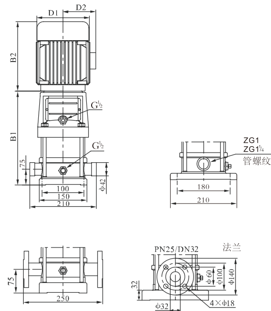
安装图
