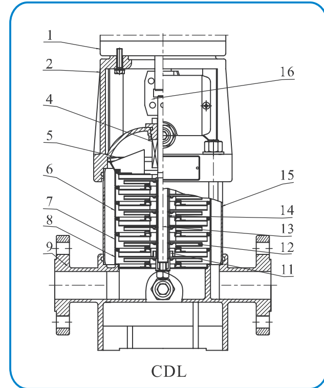
截面图 CDL,CDLF 1,2,3,4,5
