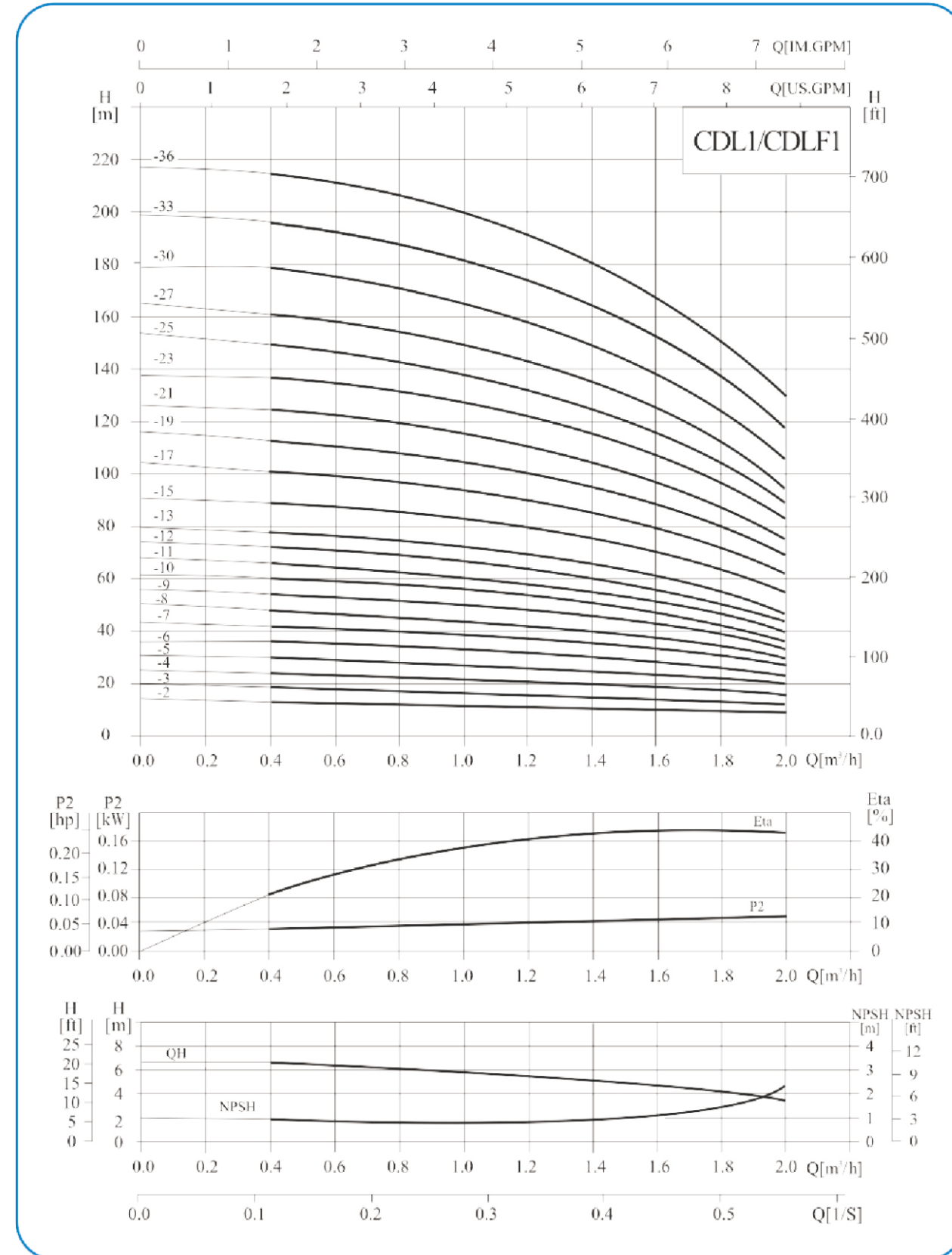
性能曲线
