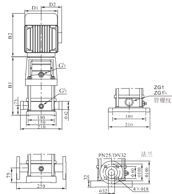
安装图
