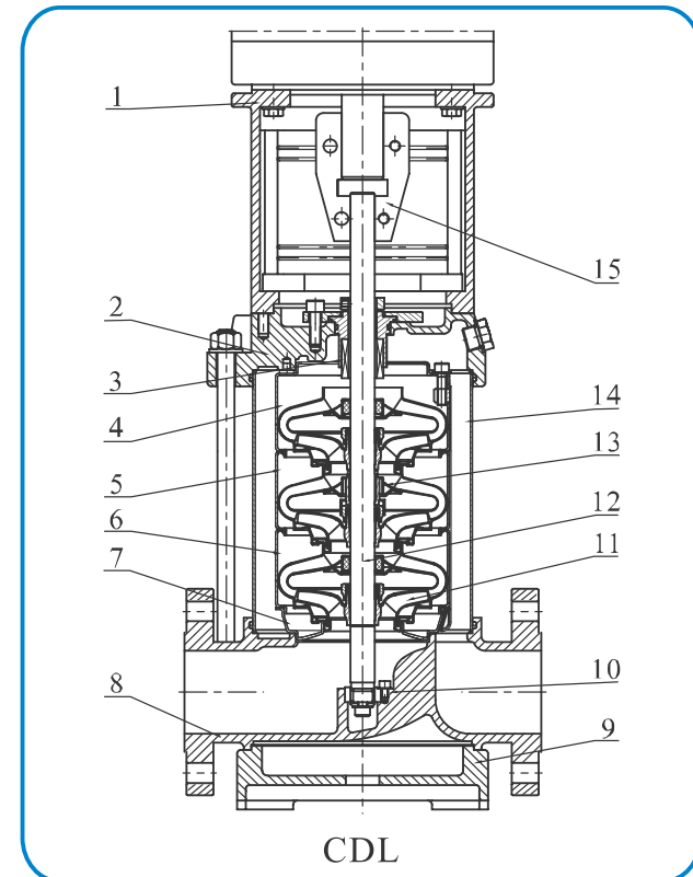
截面图 CDL,CDLF32,45,64,90
