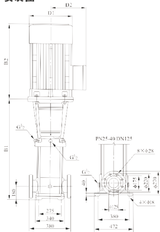
安装图
