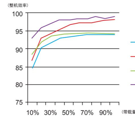
C6-10K(2014) 效率曲线示意图
