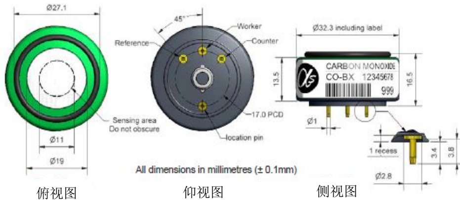
图1 CO-BX示意图
