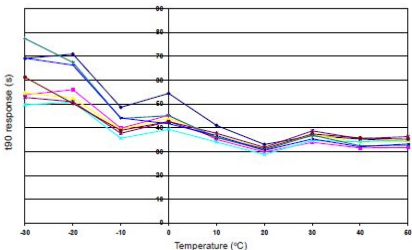
图4 响应时间的温度特性
