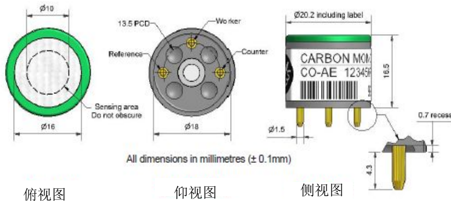
图1 CO-AE示意图
