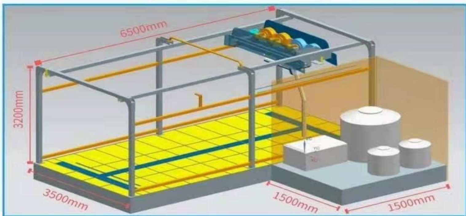
场地布局图
