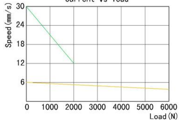
2V DC 电流与负载关系图 24V DC Current vs load
