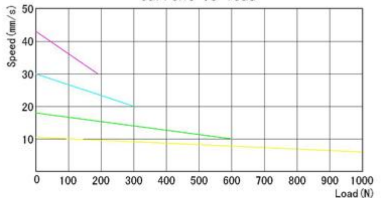
电流与负载关系图 Current vs load
