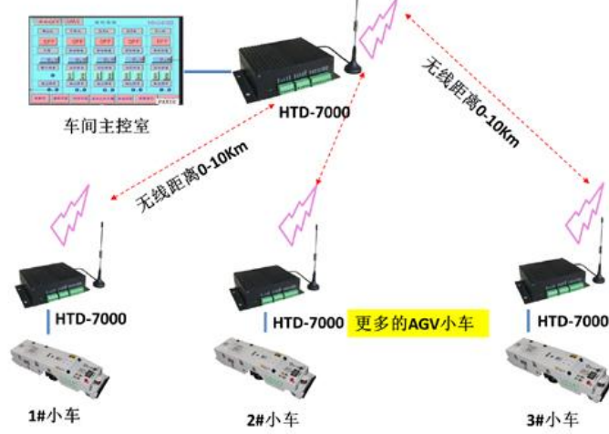
海通达HTD-7000系列工业无线开关量输出模块在AGV智能小车系统中的应用
