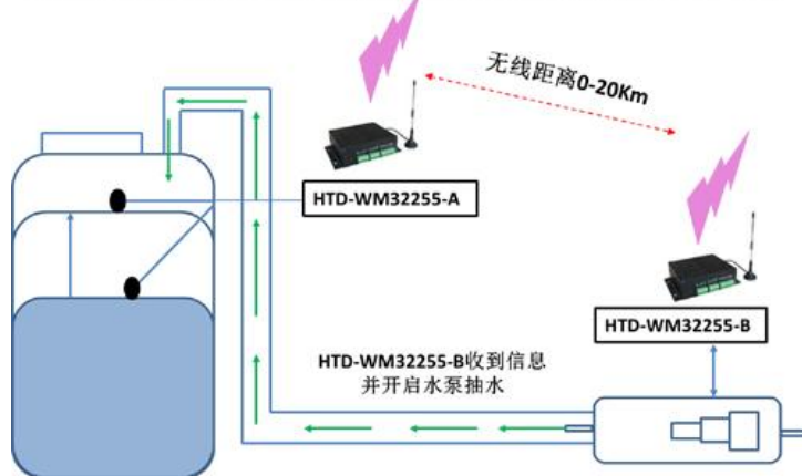
HTD-WM系列无线模拟量开关量控制器在市政供水系统中的使用（二）
