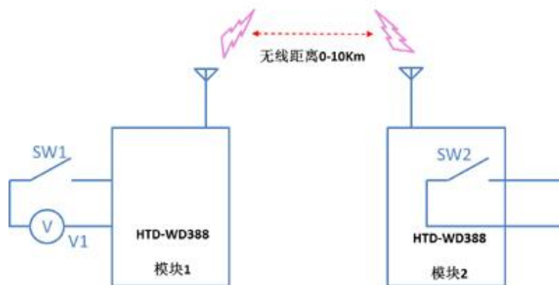
海通达HTD-WD系列无线开关量一对一使用实例
