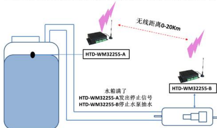
HTD-WM系列无线模拟量开关量控制器在市政供水系统中的使用（三）
