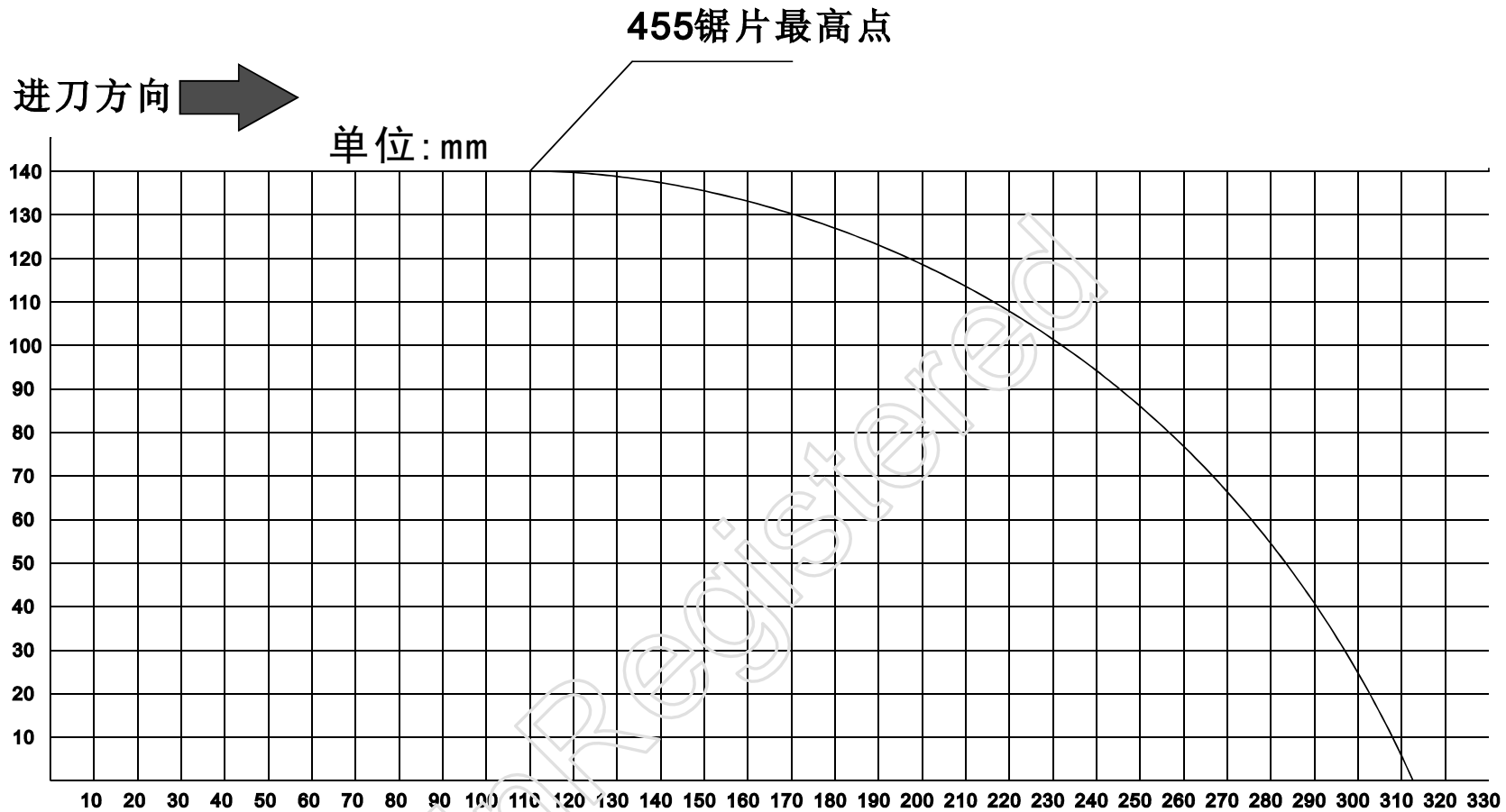
455锯片切割能力图
