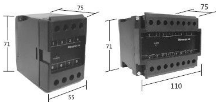
产品结构图
