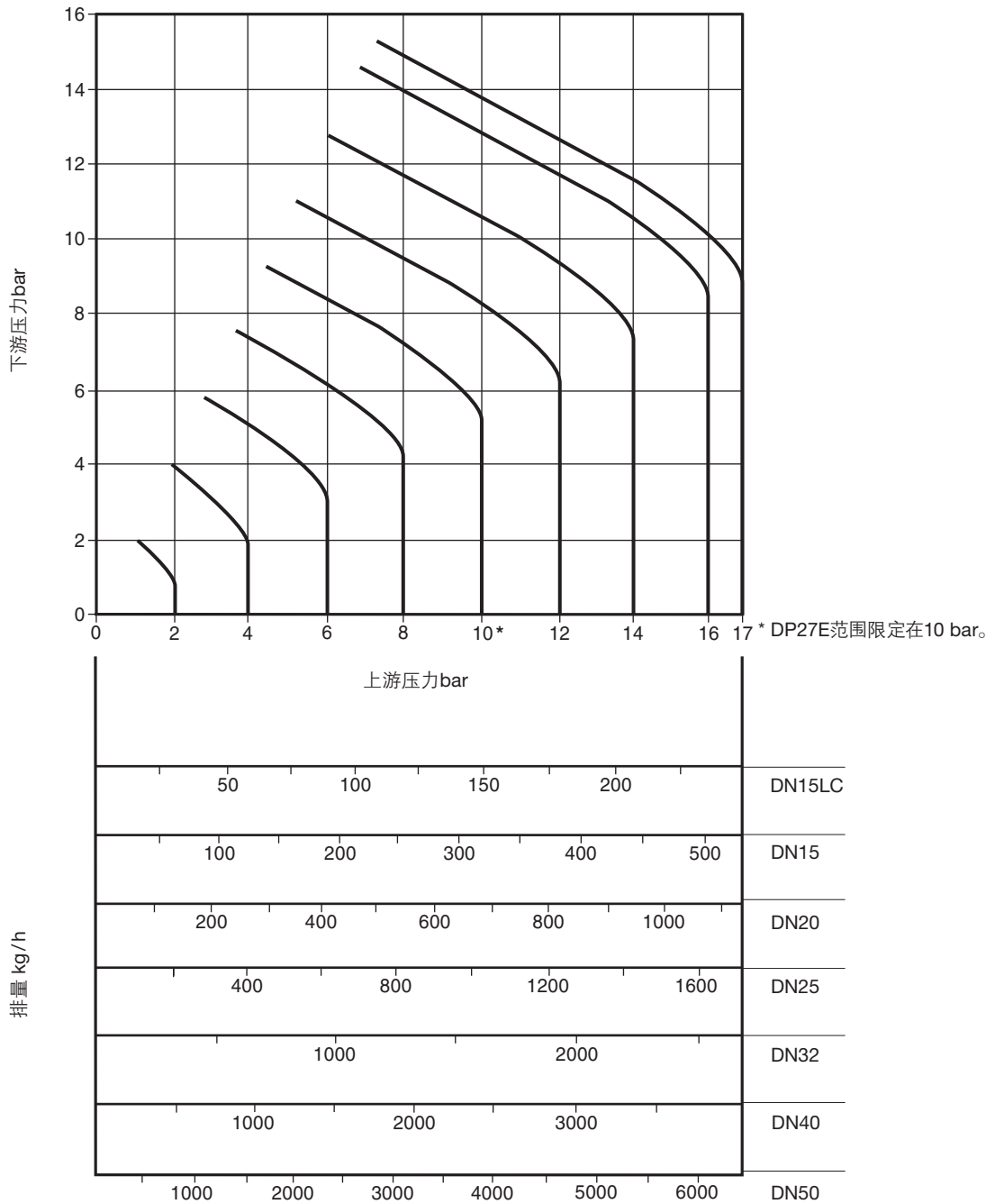
蒸汽排量图
