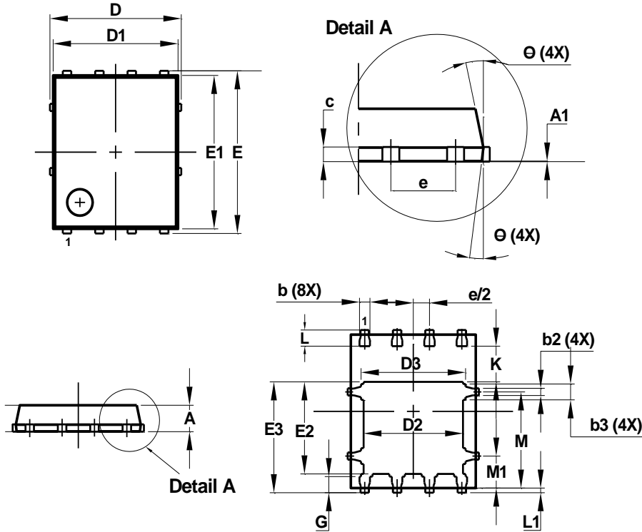
PowerDI5060-8
