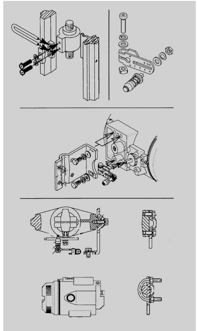
SIPART PS2 Ex d 在直行程执行机构上的安装
