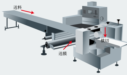
枕式包装机
