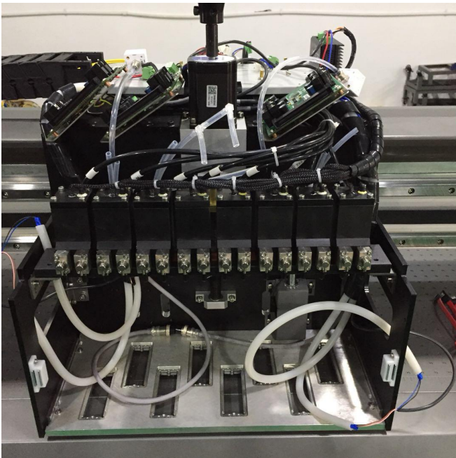
机头小车
