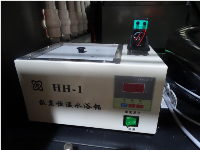
恒温控制
