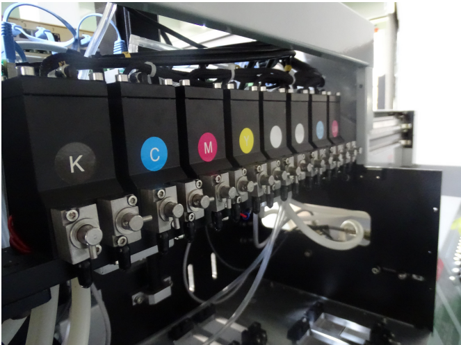
二级墨盒
