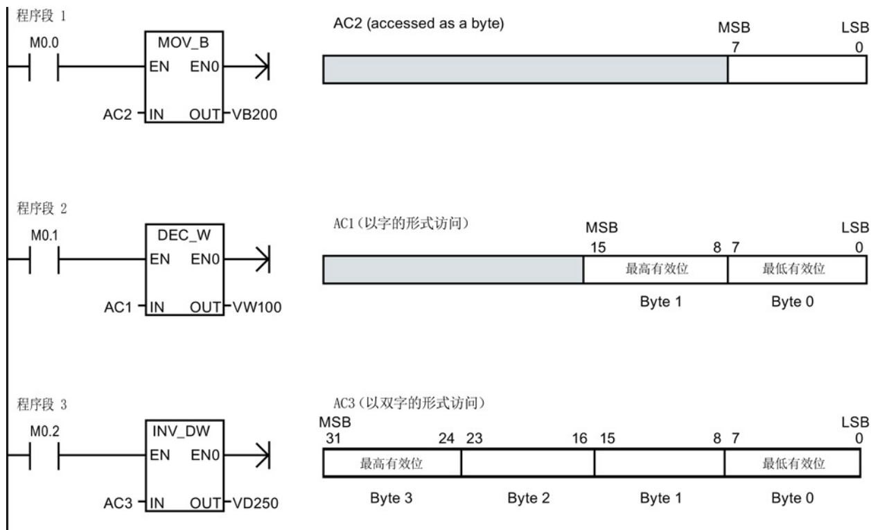
图 4-4 访问累加器
