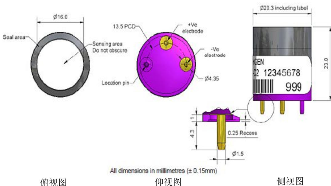
图1 O2-C2示意图
