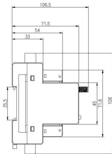
图 2 ADW300 尺寸图
