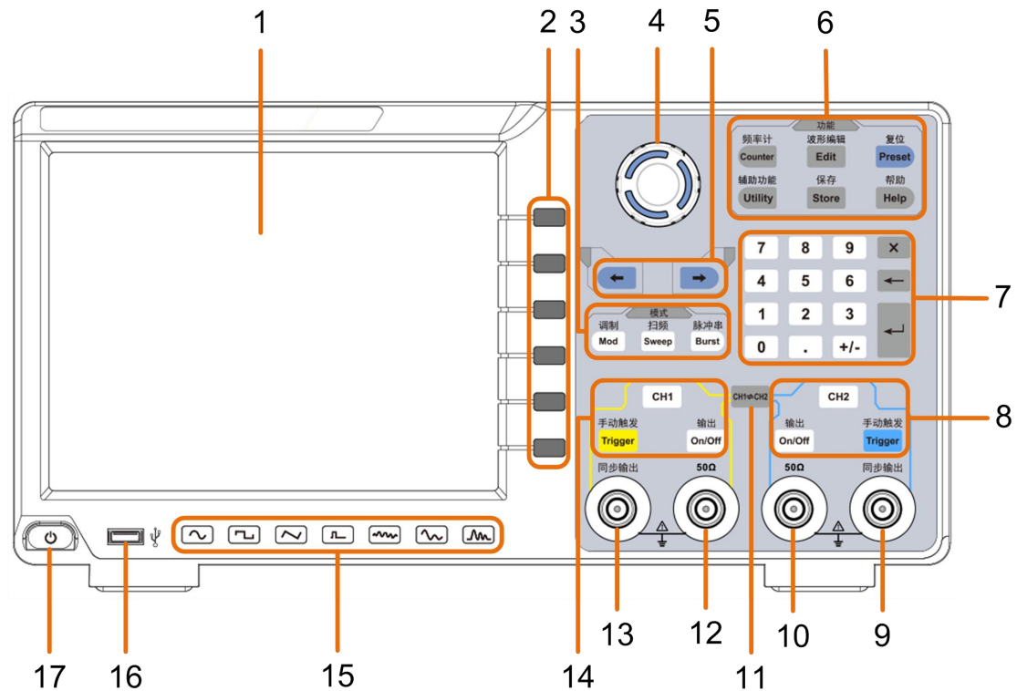
图 3-1 前面板概览
