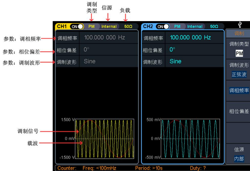
图 4-13: 相位调制的用户界面
