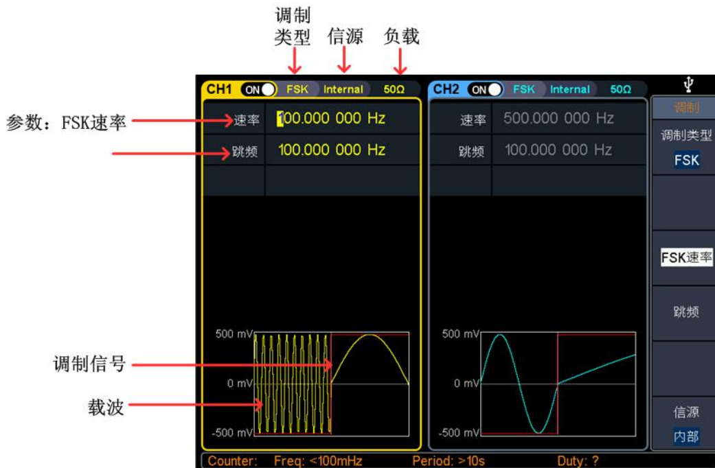
图 4-17：频移键控调制的用户界面
