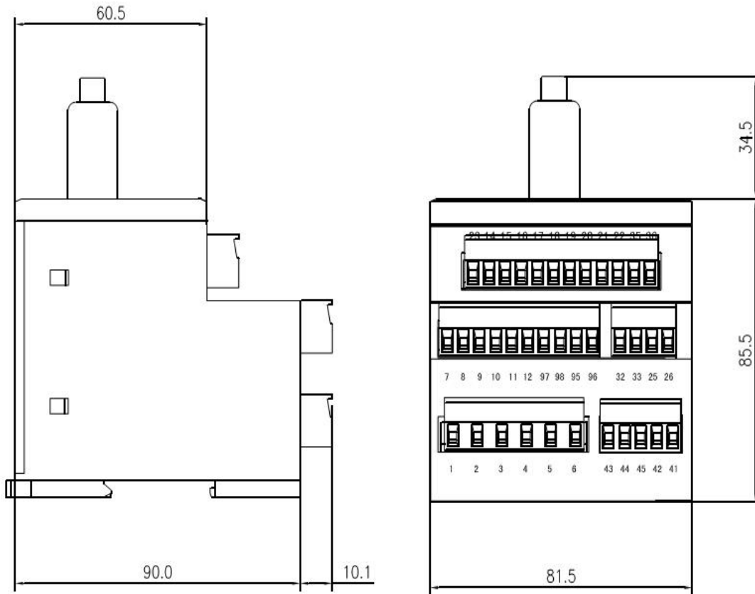
主视图
