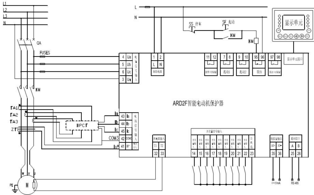
ARD2F 电动机保护器 1A、5A 规格的接线图：
