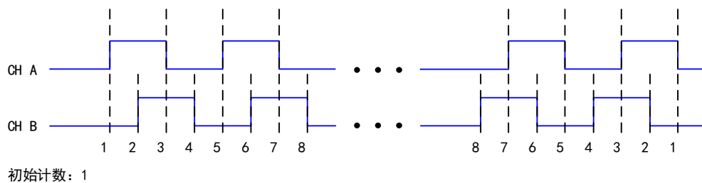
图 4-7-3 X4 编码
