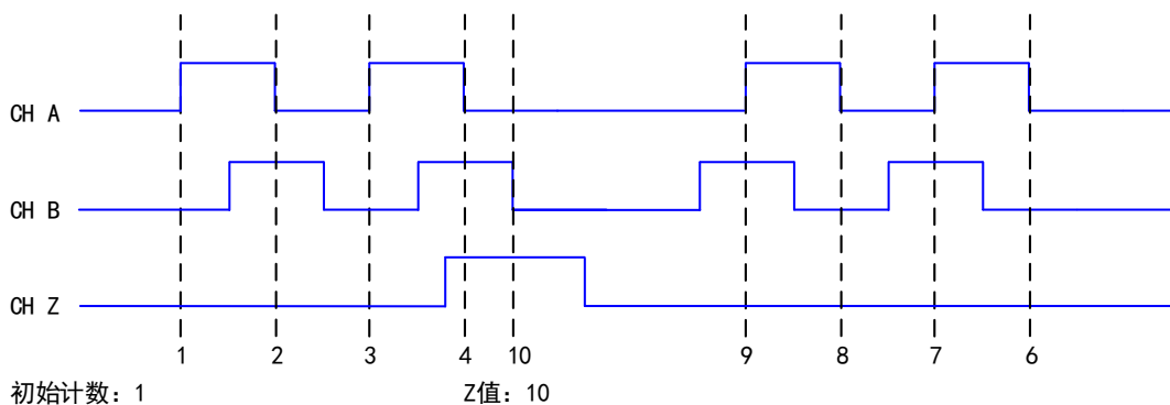
图 4-7-6 Z 索引
