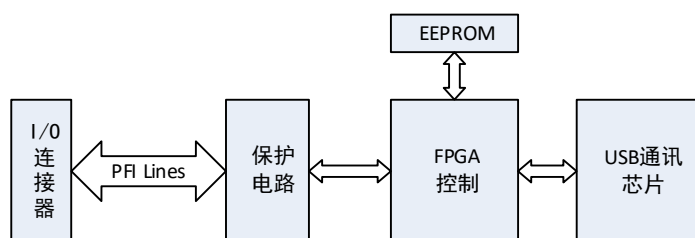
图2-2-1 USB2381_2383系统框图
