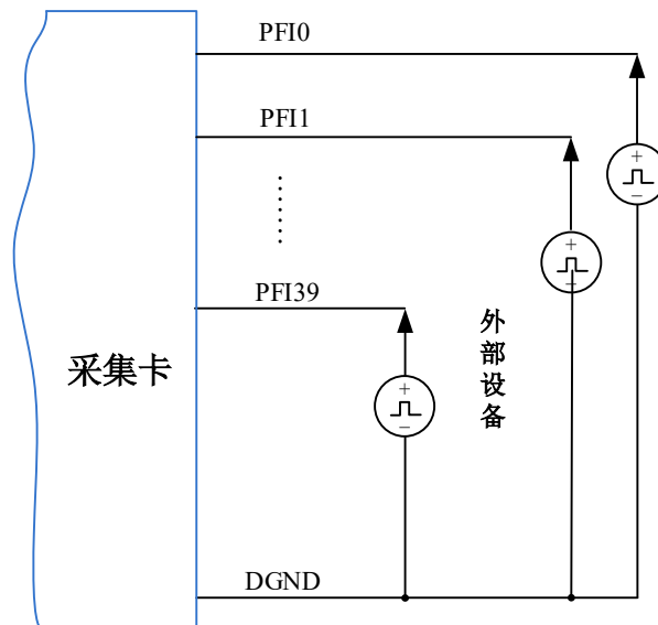
图5-2-1 DI 数字量输入的连接
