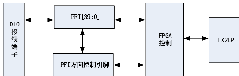
图5-1-1 DIO功能框图
