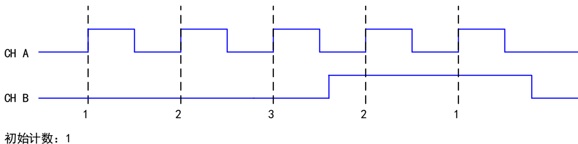
图 4-7-5 单脉冲编码
