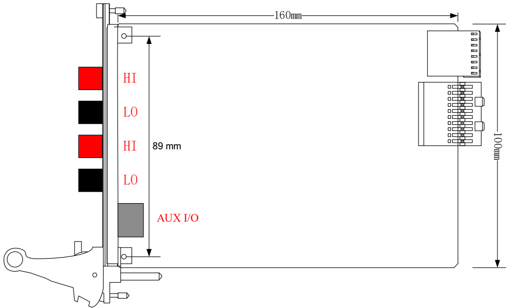
图 3-2-2 PXIe7065 板卡尺寸图
