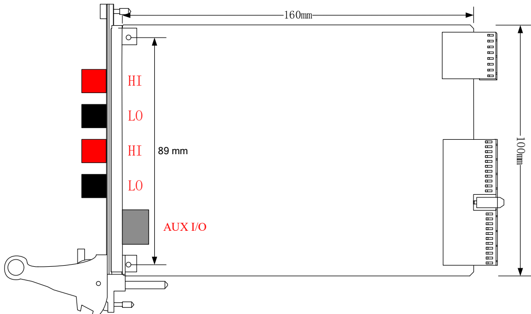
图 3-2-1 PXI7065 板卡尺寸图
