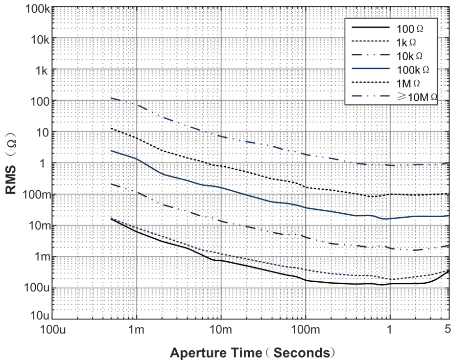
图 2-3-3 直流电压噪声
