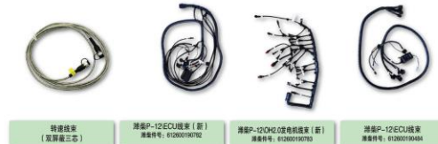
转接线束 (双屏蔽芯芯) 潍柴P-12 ECU线束(新) 产品型号: 61260190762 潍柴P-12 CH2.0发电机线束(新) 产品型号: 61260190763 潍柴P-12 ECU线束 产品型号: 61260190464
