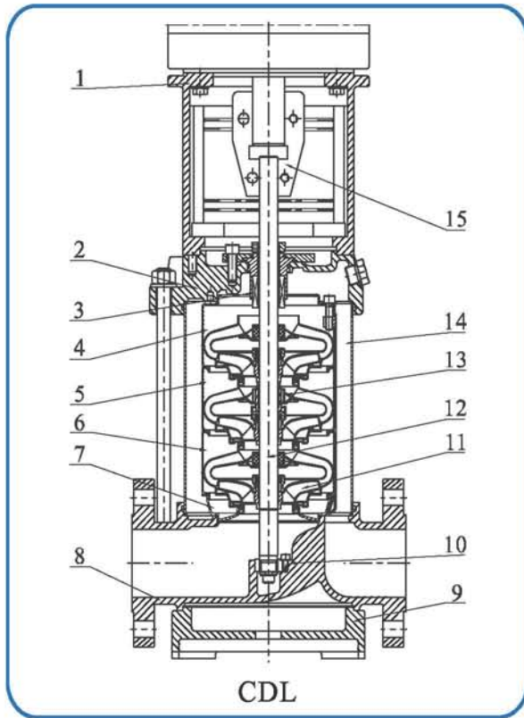
截面图 CDL,CDLF32,42,65,85
