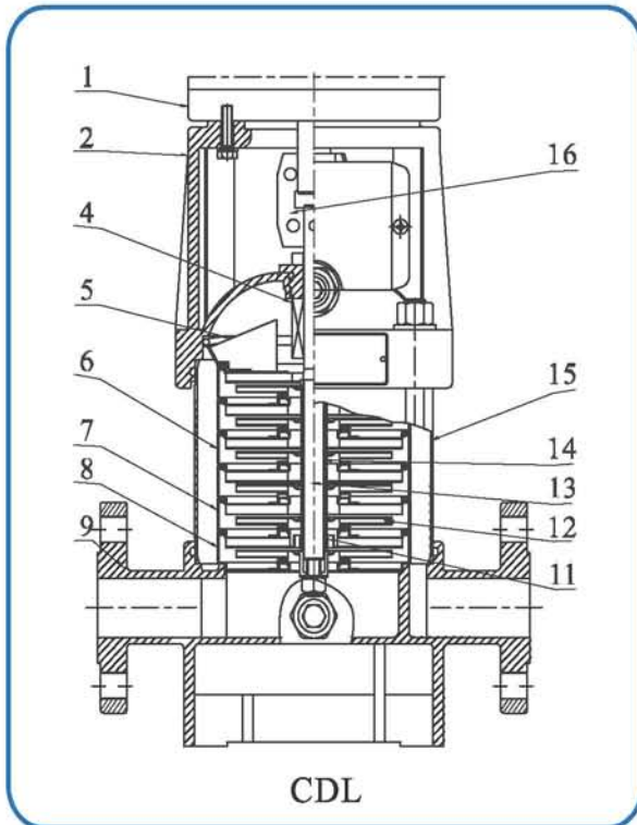
截面图 CDL, CDLF1,2,3,4,5
