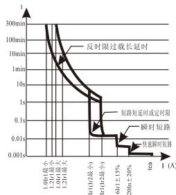
YJCPS 配电保护时间-电流特性
