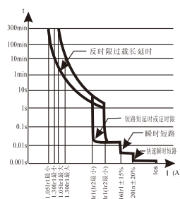
YJCPS 电动机保护时间-电流特性
