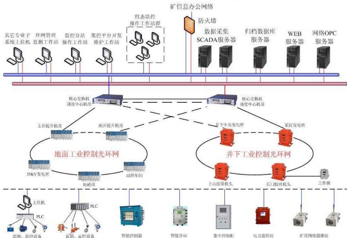
矿井工业以太环网网络平台拓扑图
