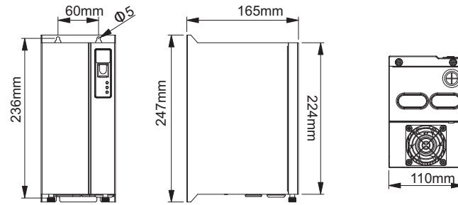
图2-8 BU制动单元外型尺寸图
