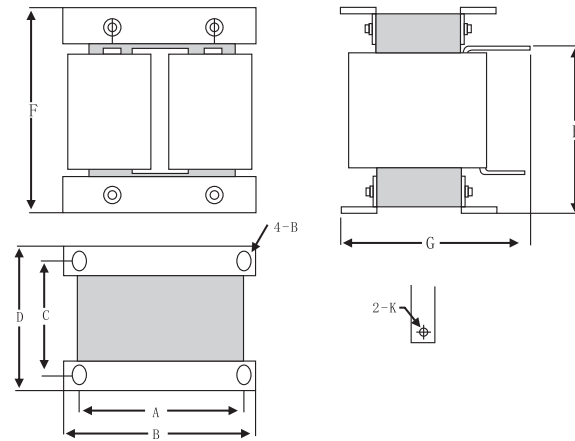
图2-7 外置电抗器尺寸示意图
