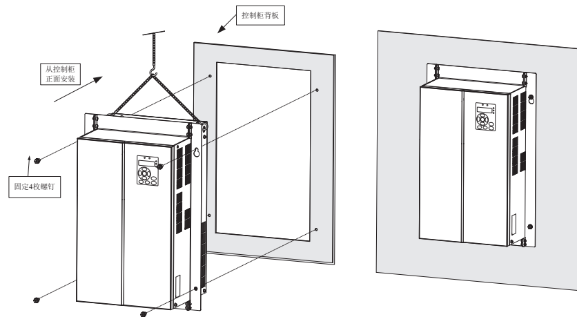
图3-10 钣金结构嵌入式安装示意图
