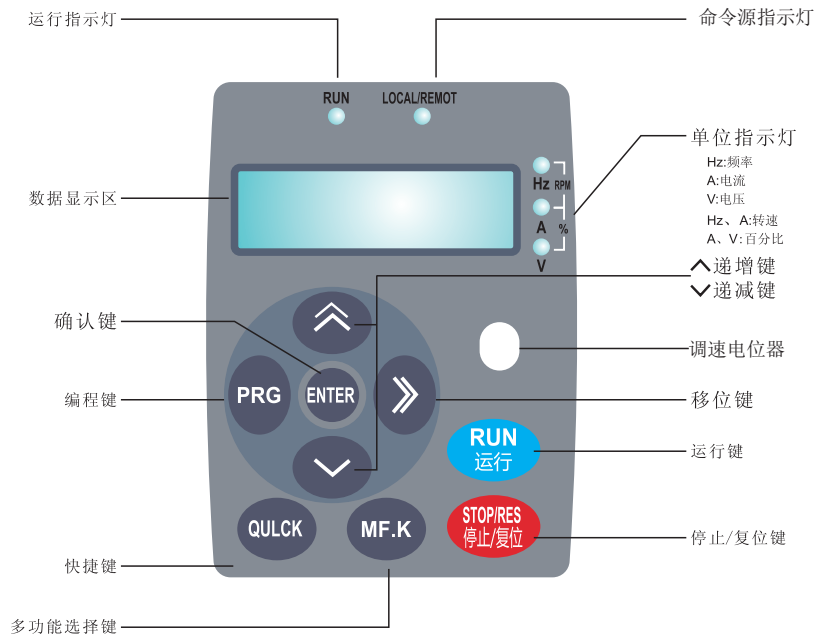
图4-2带电位器的外引键盘示意图
