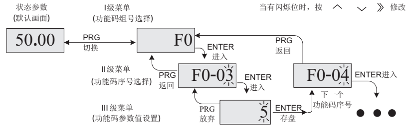
图4-3 三级菜单操作流程图
