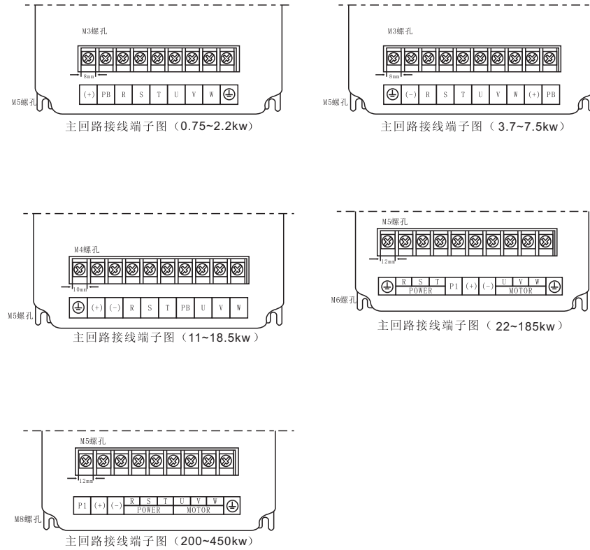
图3-14 变频器主回路端子分布
