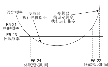
图5-44 休眠与唤醒延迟时间
