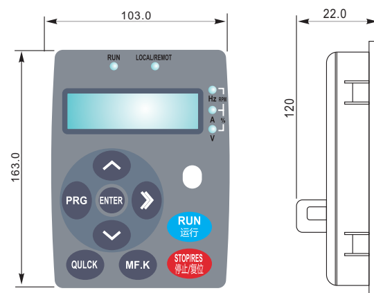
图2-5 外引键盘的外型尺寸 (单位: mm)
