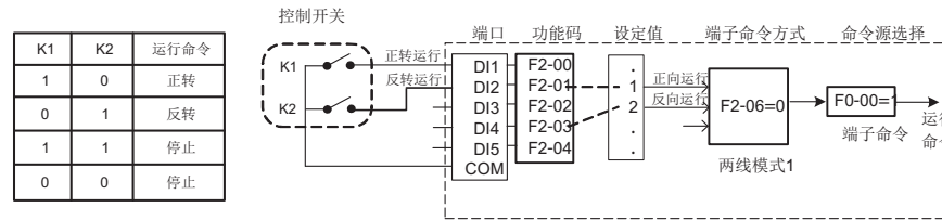
图5-5 两线式模式1
