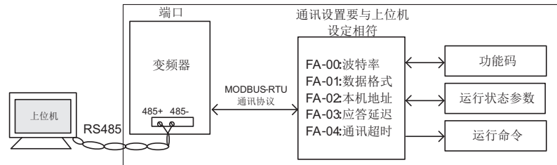
图3-24 变频器串行通讯的使用
