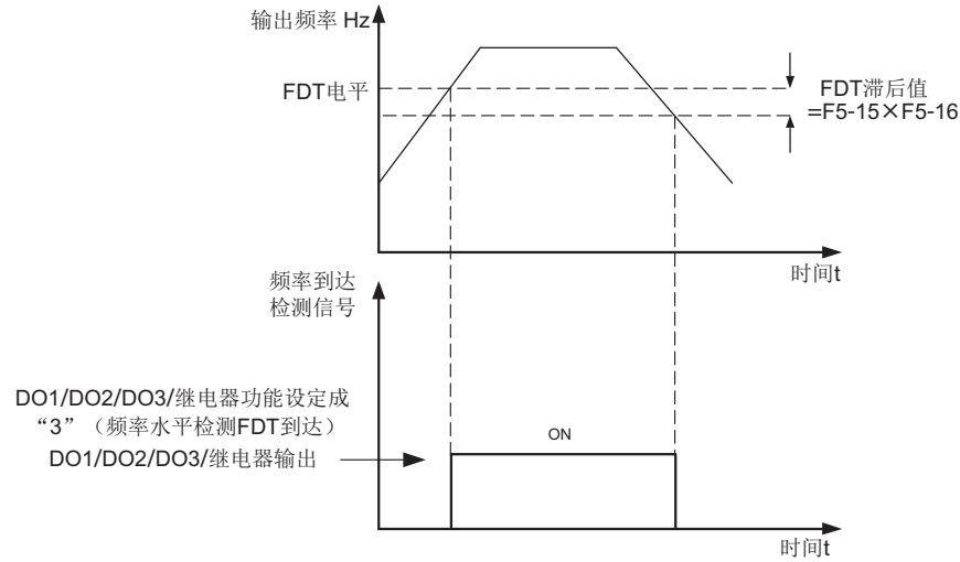
图5-42 FDT电平检测示意图
