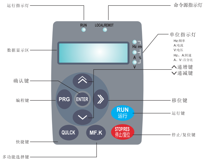
图4-1操作面板示意图
