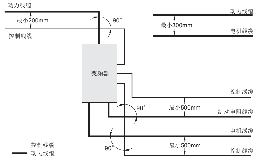
图6-5 电缆布线图
