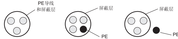
图6-2 带屏蔽层的屏蔽电缆
