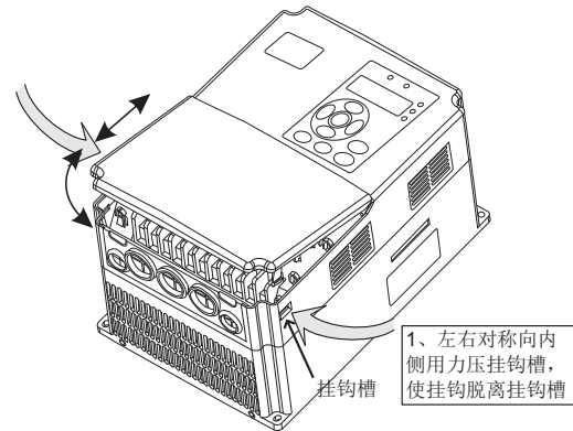
图3-12 塑胶外壳下盖板拆卸图
