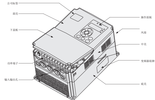
图2-1 变频器塑胶结构外型图
