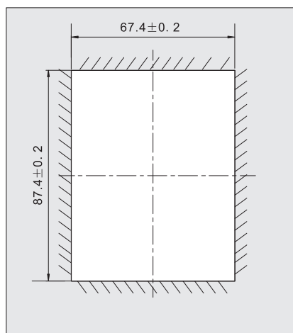
图2-6 外引键盘安装开孔示意图
