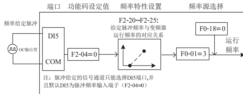
图5-12 脉冲给定频率功能码设置
