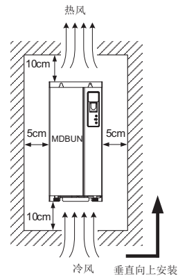
图2-9 BU制动单元的安装间距
