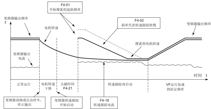
图5-39 转速跟踪再启动
