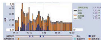
显示耗电量履历和运转状态
