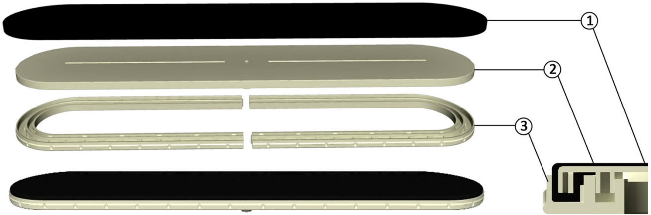
装配图
