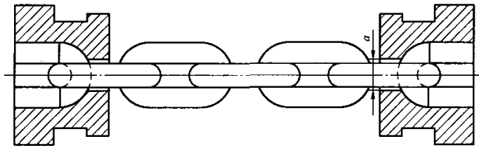
图3 链条固定装置
