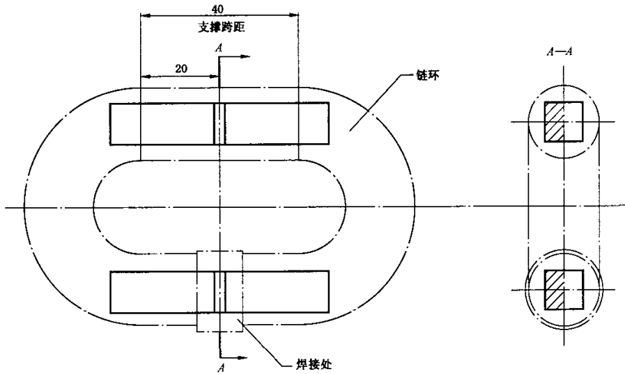
图 C.1 缺口冲击试验试件
