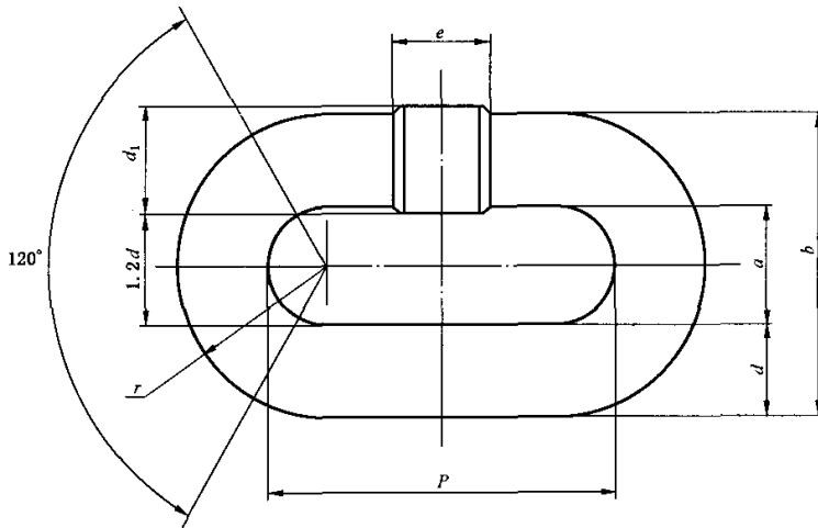
图 2 链环尺寸
