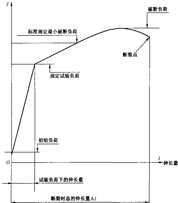
图 5 静拉伸曲线
