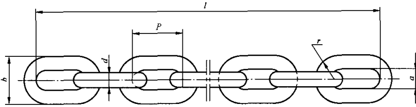
图 1 链条型式和尺寸
