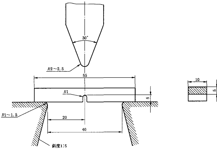
图 C.2 夏比冲击试验(U形缺口)尺寸
