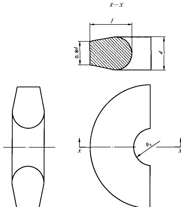
图4 插入销外形
