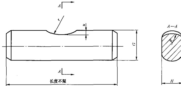
图6 固定销
