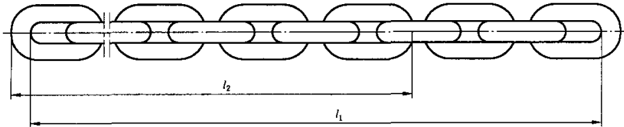
图 B.1 链条配对长度
