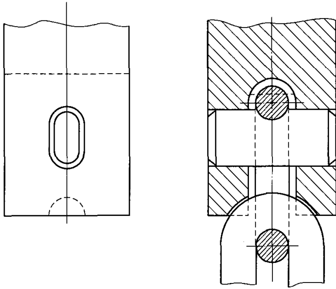
图7 固定叉头
