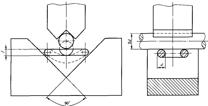
图8 弯曲试验
