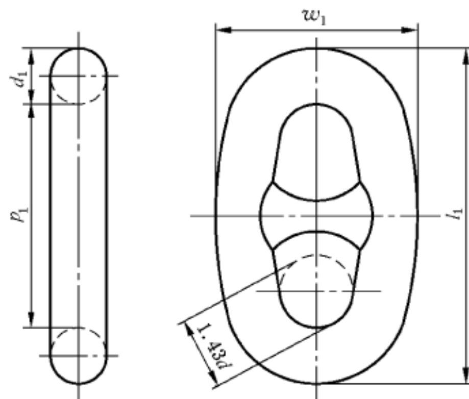
图 4 加大链环
